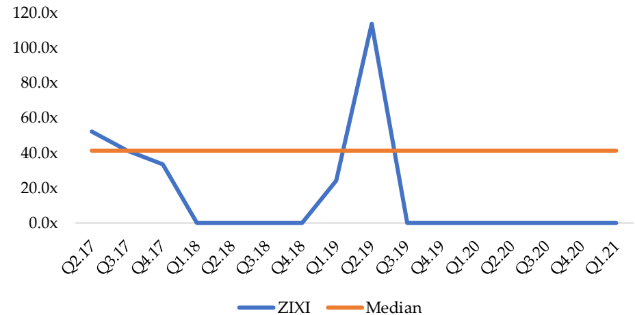
P/E Zix
