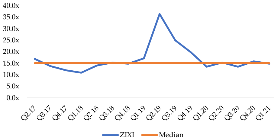
EV/EBITDA Zix
